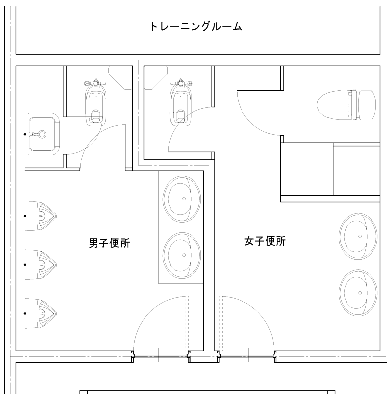
中 2 階 平面詳細図 S : 1/50
