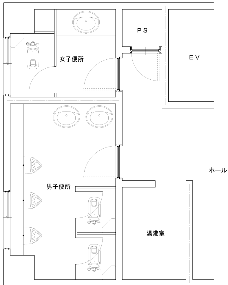
5階 平面詳細図 S : 1/50
