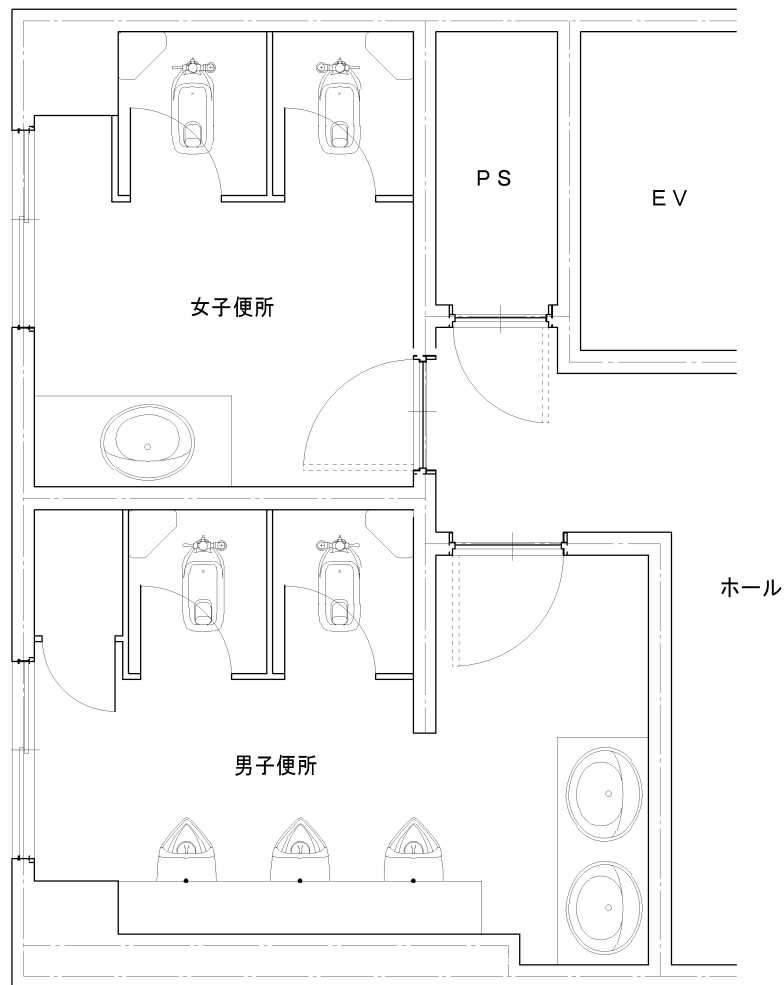
2 ~ 4 階 平面詳細図 S : 1/50
